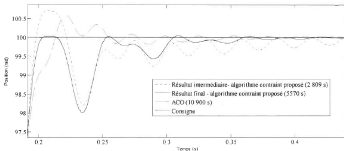
Figure 4-19 Agrandissement de la réponse à l'échelon pour le contrôleur pondéré PID_F avec un retour d'anti-saturation sur le courant.
