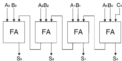
Figure 4.10 : Schémas du CSA (a) et du RCA (b) 4bits.
