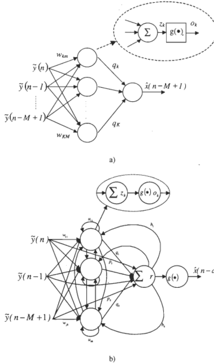
Figure 3.7 : Les réseaux de neurones PL-MNN (a) et PL-RNN (b).
