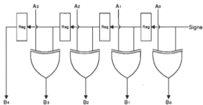
Figure 4.12 : Schéma du complément à 1.
