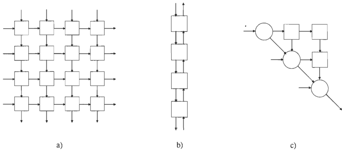
Figure 4.3 : Exemples d'architectures systoliques
