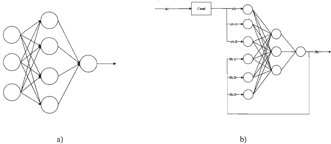
Figure 3.5 : Schématisation d'un RNA multicouche (a) et d'un RNA récurrent (b) (NARX).
