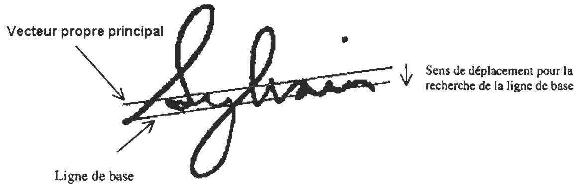
Figure 4.11 : Recherche de la ligne de base.
