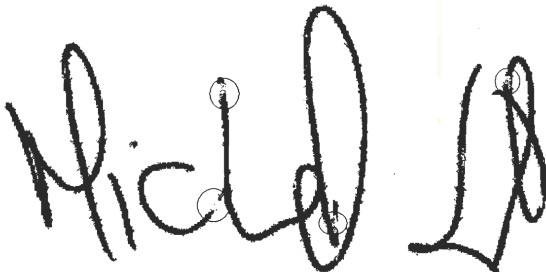
Figure 3.2 : Binarisation brut.
