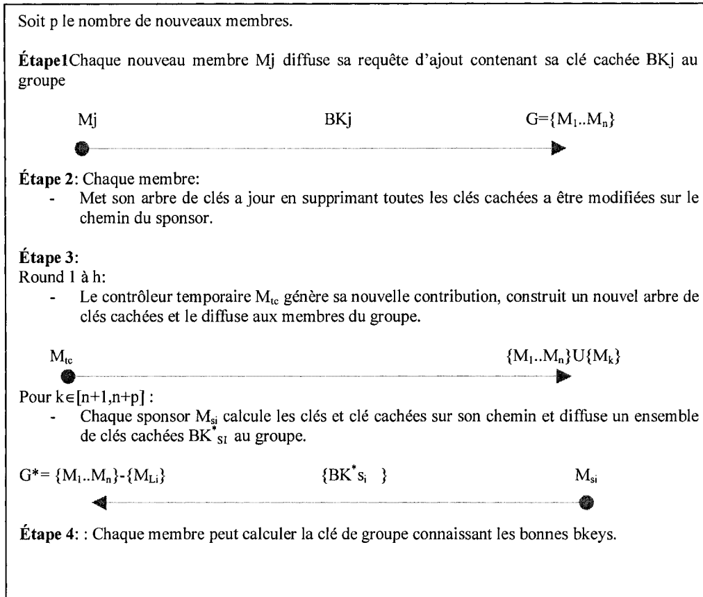
Figure 30: Interaction lors du protocole d'ajout multiple.
