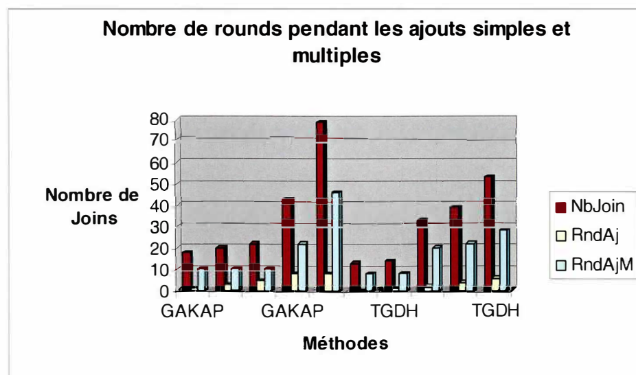
Figure 35 : Nombre de rounds à la suite des ajouts simples et multiples
