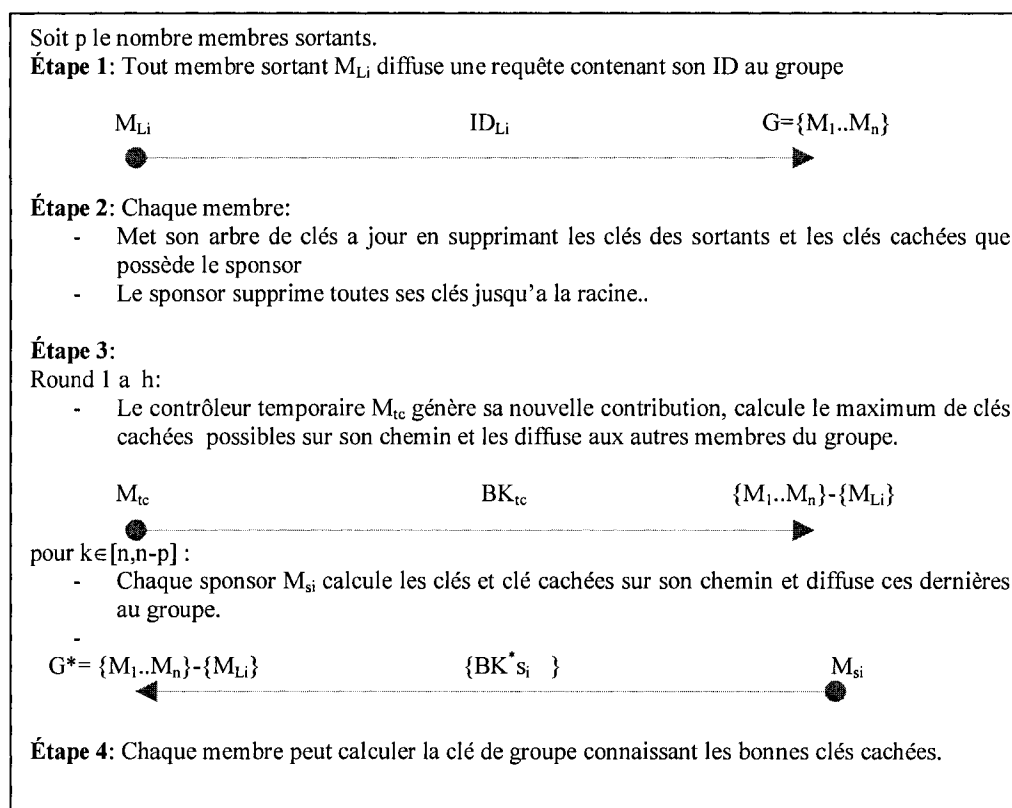
Figure 31: Interaction lors du départ multiple
