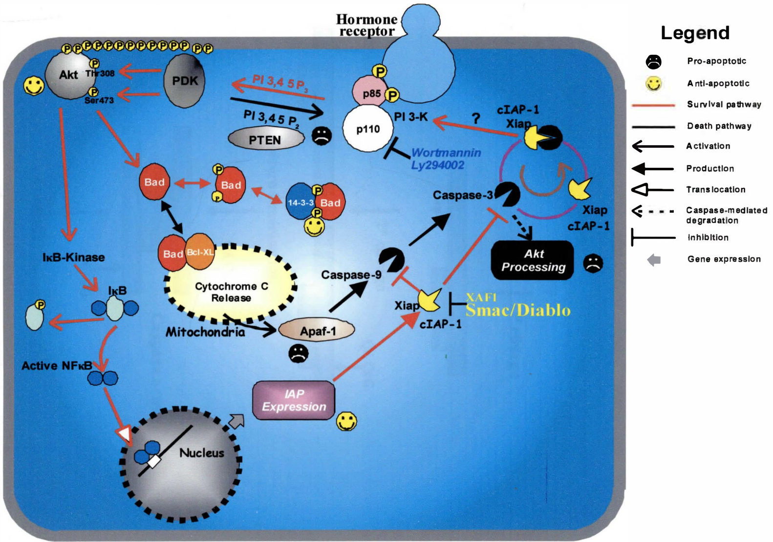
FIGURE 1.8 : Représentation schématique des voies de signalisation cellulaire impliquées lors de processus pro-apoptotiques et/ou anti-apoptotiques.
