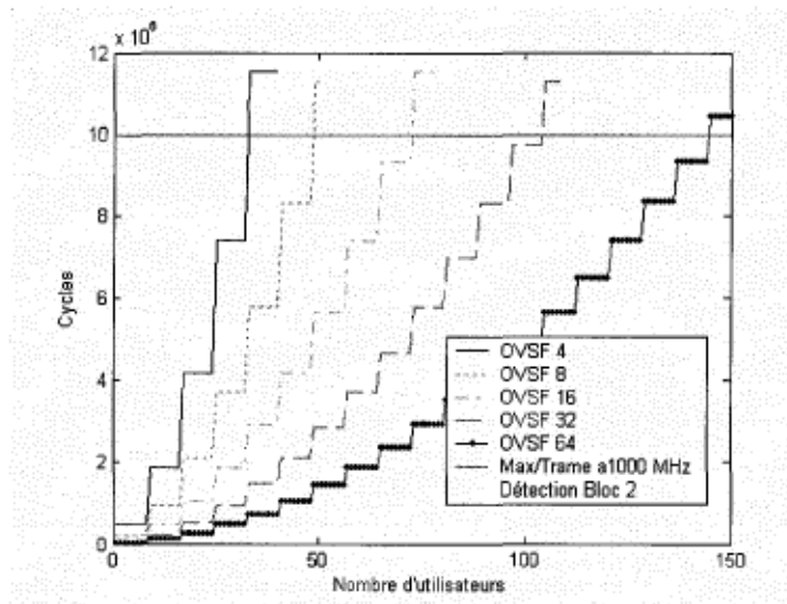
Figure 5.6 Détection du bloc Détection avec N_{\text{chips}}=38400 , N_v=3U , f=1\text{GHz} .
