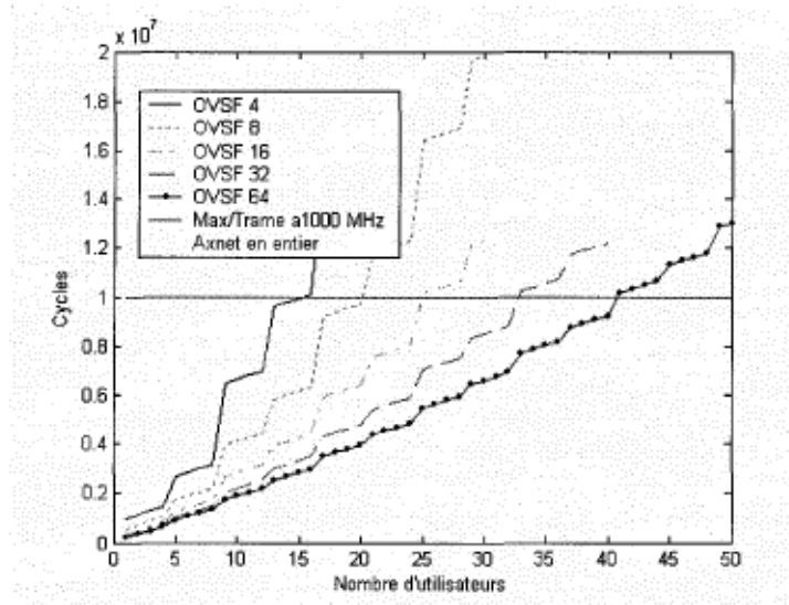
Figure 5.9 CF-MUD en entier (version assembleur) avec N_{\text{chips}}=38400 , N_{\text{adapt\_chips}}=256 \cdot 100/\text{OVSF} , N_w=2 \cdot \text{OVSF} , N_v=3U , f=1\text{GHz} .
