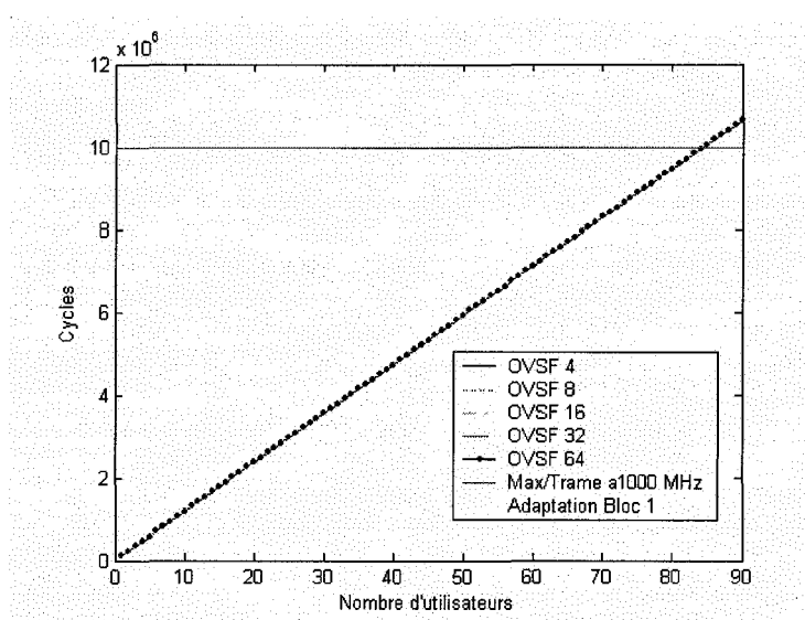
Figure 5.3 Adaptation du bloc Signature avec N_{\text{adapt\_chips}} = 256 \cdot 100 / \text{OVSF} , N_w = 2 \cdot \text{OVSF} , f = 1 \text{ GHz} .
