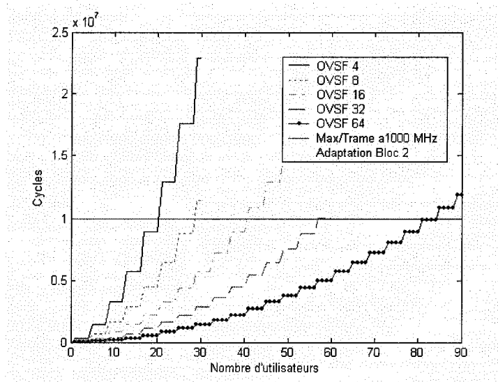
Figure 5.5 Adaptation du bloc Détection avec N_{\text{adapt\_chips}} = 256 \cdot 100 / \text{OVSF} , N_v = 3U , f = 1\text{GHz} .
