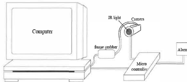
Figure 2.3: Les composantes matérielles utilisées [1].
