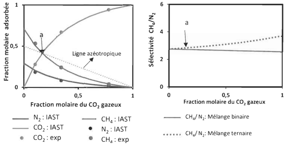
Figure 13 Adsorption du mélange ternaire CO 2 /CH 4 /N 2 sur le MOF-5 à pression constante (1500 kPa) ; la fraction molaire du CO 2 dans la phase gazeuse varie de 0 à 1 tandis que celles des autres constituants sont égales.
