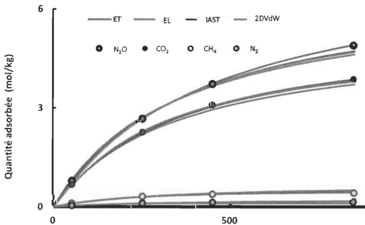
Figure 16 Adsorption du mélange quaternaire N_2O-CO_2-CH_4-N_2 sur le CuBTC à 297 K
