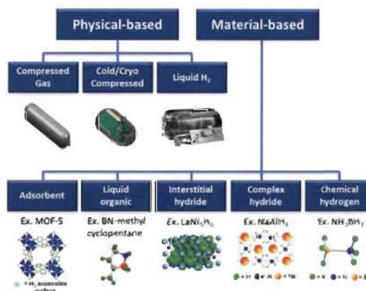
Figure 1.3 : Systèmes de stockage d'hydrogène [11].
