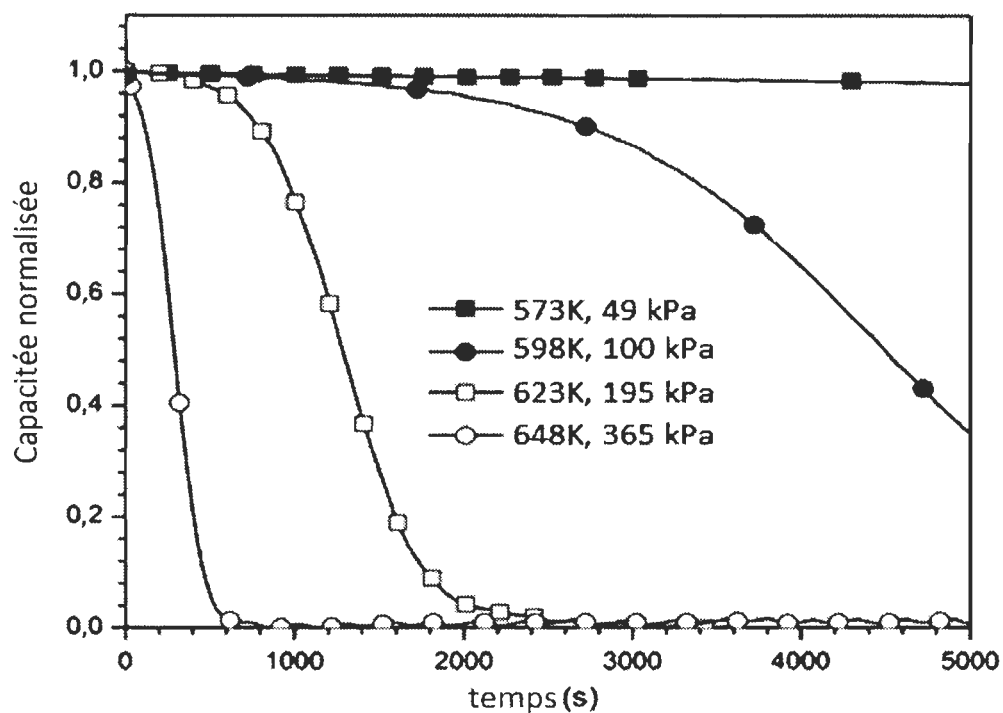
Figure 24 - Cinétiques d'absorption et de désorption à différentes températures avec une force motrice constante
