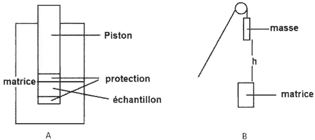
Figure 7 - Schématique du forgeage
