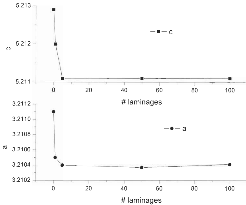
Figure 14 - Paramètres de maille du magnésium en fonction du nombre de laminages
