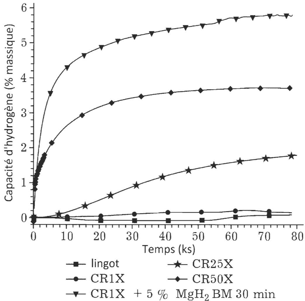
Figure 15 - Cinétique d'activations de différents échantillons de magnésium à 2 MPa et 623K
