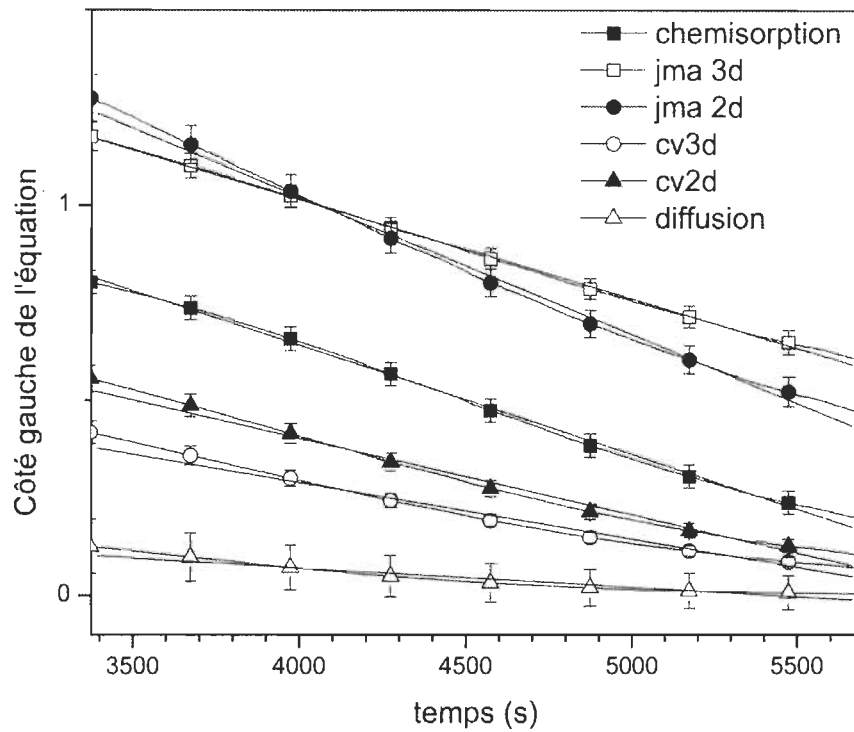
Figure 31 - Courbes de calculs d'étape limitative du cœur de la désorption à 598 K ainsi que leur régression linéaire
