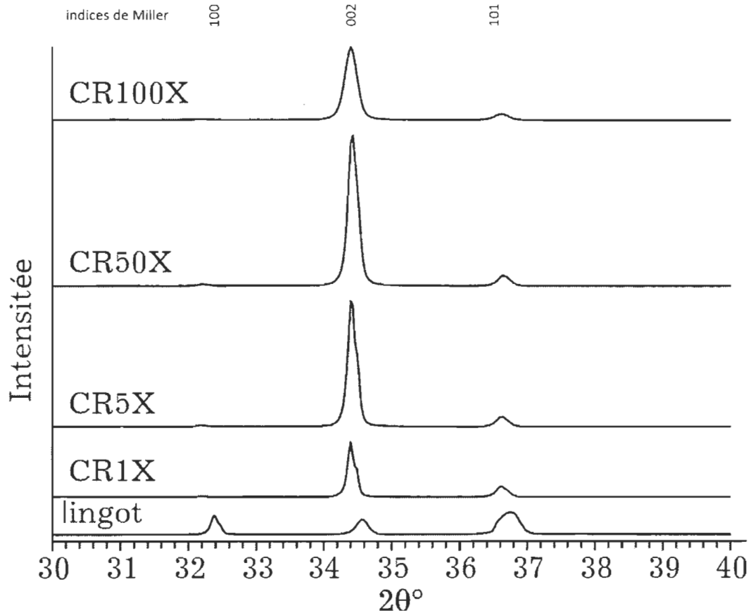
Figure 13 - Diffractogrammes X du magnésium en lingot ainsi que laminé 1, 5, 50 et 100 fois.
