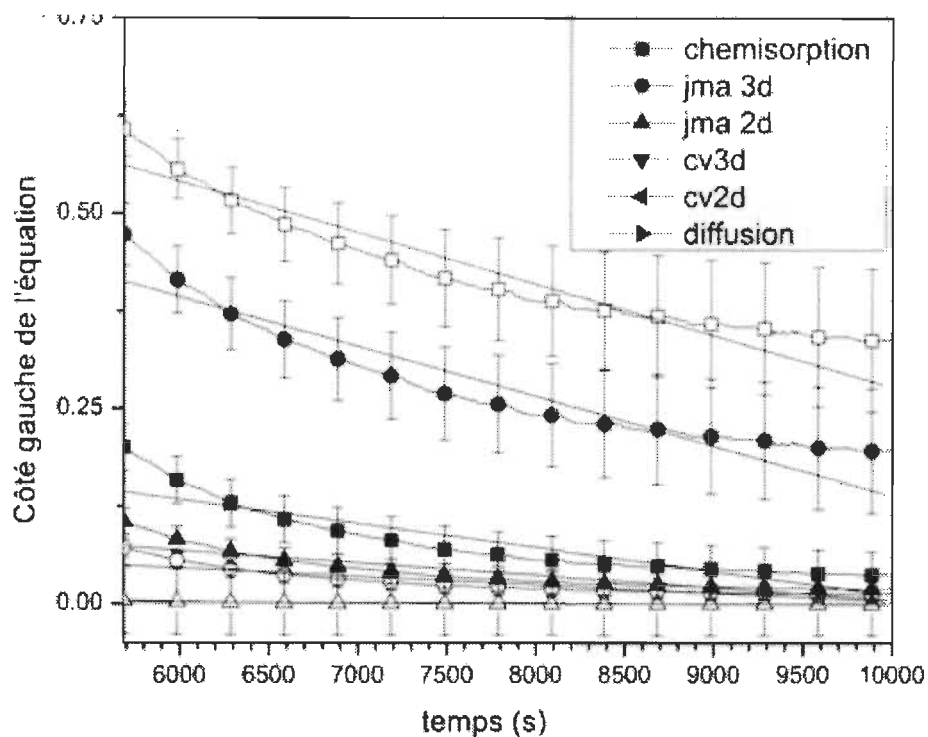
Figure 32 - Courbes de calculs d'étape limitative de la fin de la désorption à 598 K ainsi que leur régression linéaire
