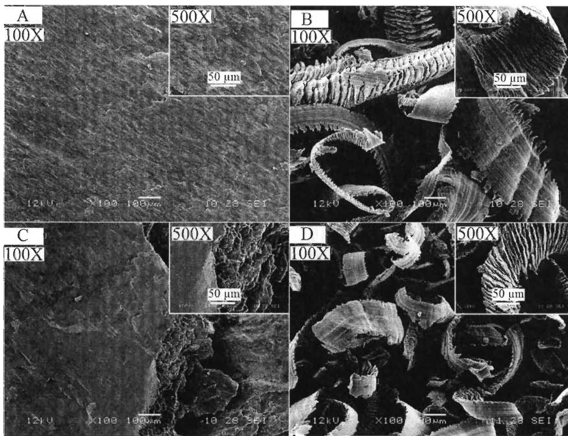
Figure 35 - Images MEB: A – Mg laminé, B – Mg limé, C – Mg limé et ensuite laminé, D – Mg laminé et ensuite limé.
