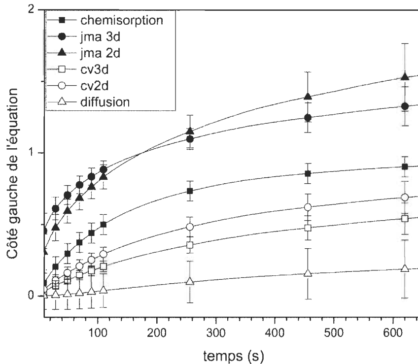
Figure 27 - Courbes de calculs d'étape limitatives d'absorption à 598 K ainsi que leur régression linéaire calculée entre 10 et 90 % de la complétion de la réaction
