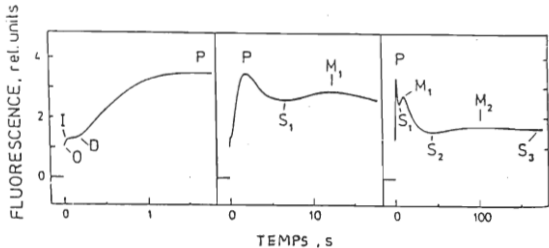
Figure 14. Fluorescence variable mesurée sur différentes échelles de temps avec l'inscription des transients caractéristiques.
