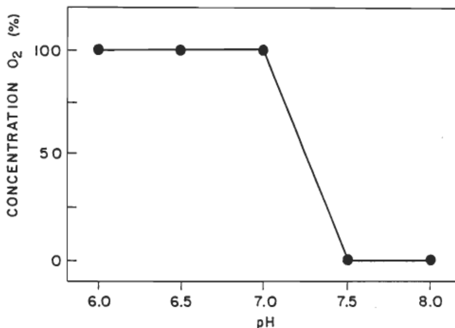
Figure 23. Effet du pH sur la concentration d'oxygène en solution en présence de 10 mM sulfite de sodium.
