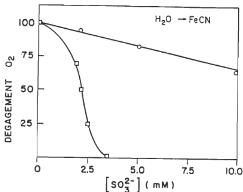
Figure 25. Comparaison de l'activité mesurée en présence de sulfite et en absence de sulfite dans la suspension de chloroplastes.
