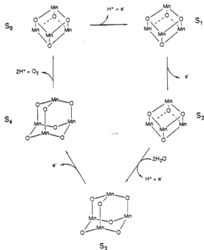
Figure 13. Modèle de coordination des atomes de manganèse par les atomes d'oxygène pendant l'oxydation de l'eau. Les protons ne sont pas insérés dans le modèle.
