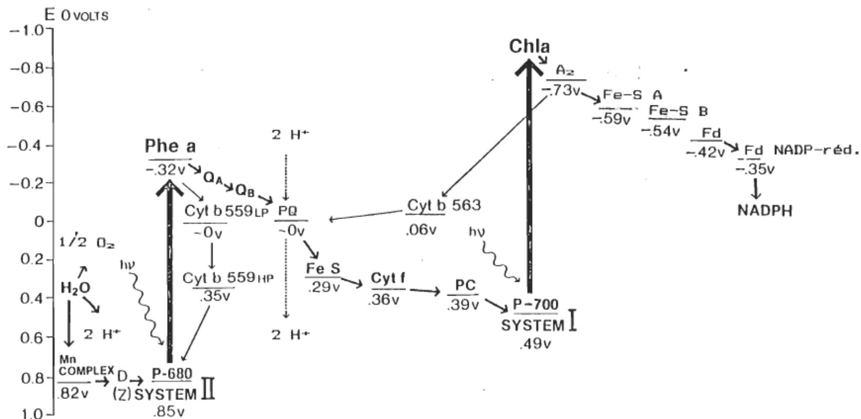
Figure 6. Schéma en Z indiquant les potentiels d'oxido-réduction au point milieu pour les composantes du transport d'électrons du thylacoïde.
