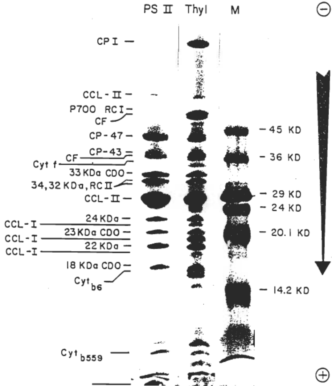
Figure 19. Séparation des protéines des chloroplastes brisés (thyl) et des MEPSII (PSII). La bande de droite est composée de protéines contrôles.
