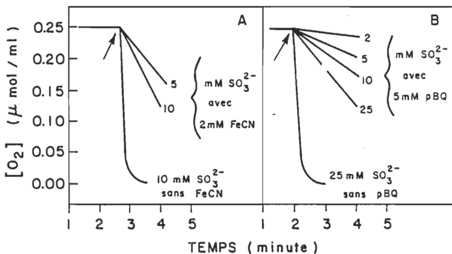
Figure 22. Effet du sulfite sur la concentration de l'oxygène en solution en présence ou non d'accepteurs exogènes. La flèche indique le moment de l'addition du sulfite de sodium.
