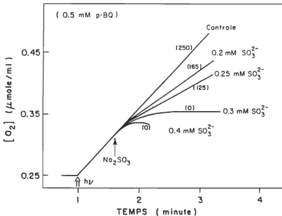
Figure 21. Effet du sulfite de sodium sur le dégagement d'oxygène des thylacoïdes. La flèche ouverte indique le début de l'illumination. La flèche noire indique le moment de l'addition du sulfite de sodium.
