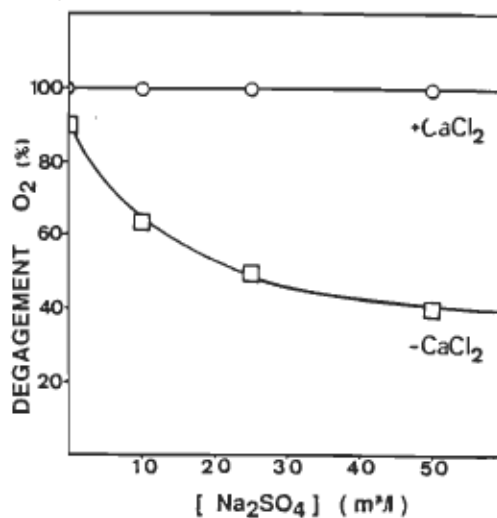
Figure 30. Inhibition de l'activité du PSII par le sulfate de sodium sous illumination.
