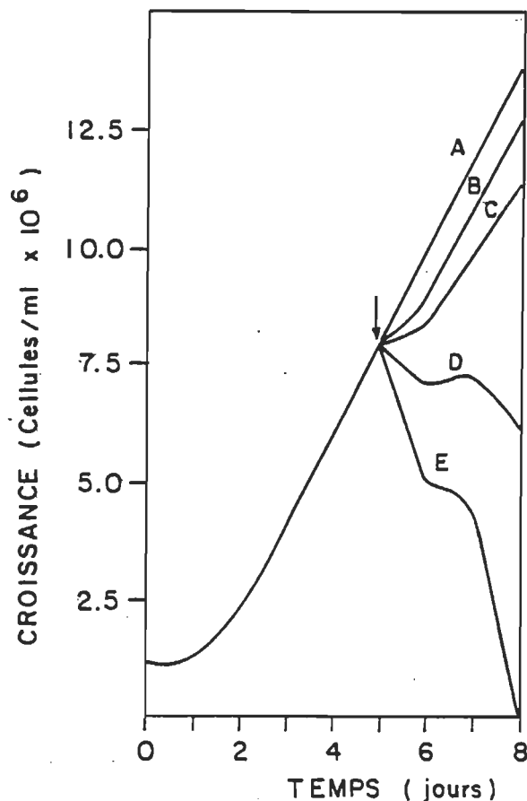
Figure 42. Effet de la concentration en sulfate sur la croissance des algues Dunaliella bardawil .
