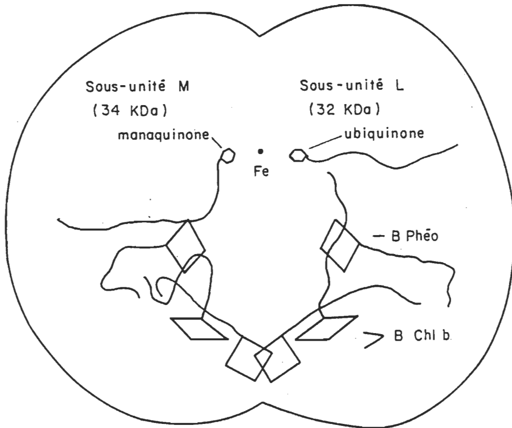
Figure 9. Centre réactionnel de Rhodospseudomonas viridis (d'après Deisenhofer et coll. 1985).
