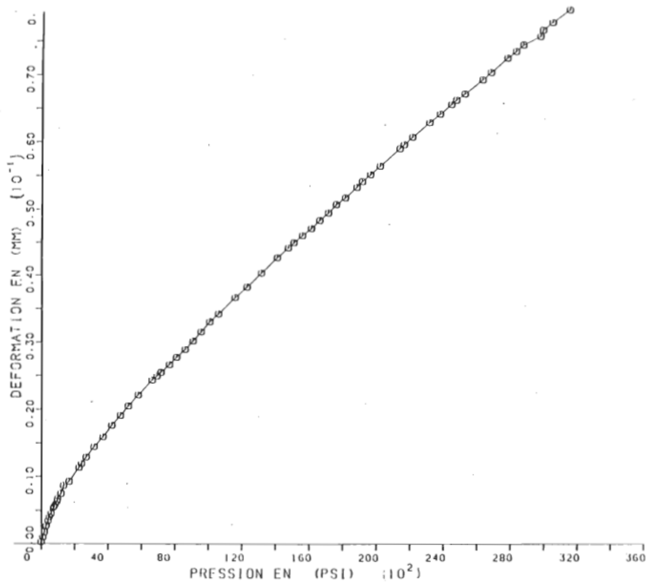
Figure (2.2): Courbe de la déformation mécanique de la cellule optique en fonction de la pression.
