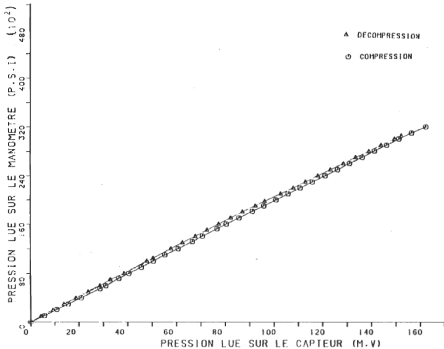
Figure (2.1) : Courbe de calibration du capteur de pression à l'aide d'un manomètre.
