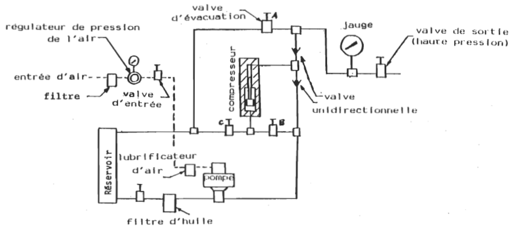
Figure (3.6) Schéma de fonctionnement du compresseur
