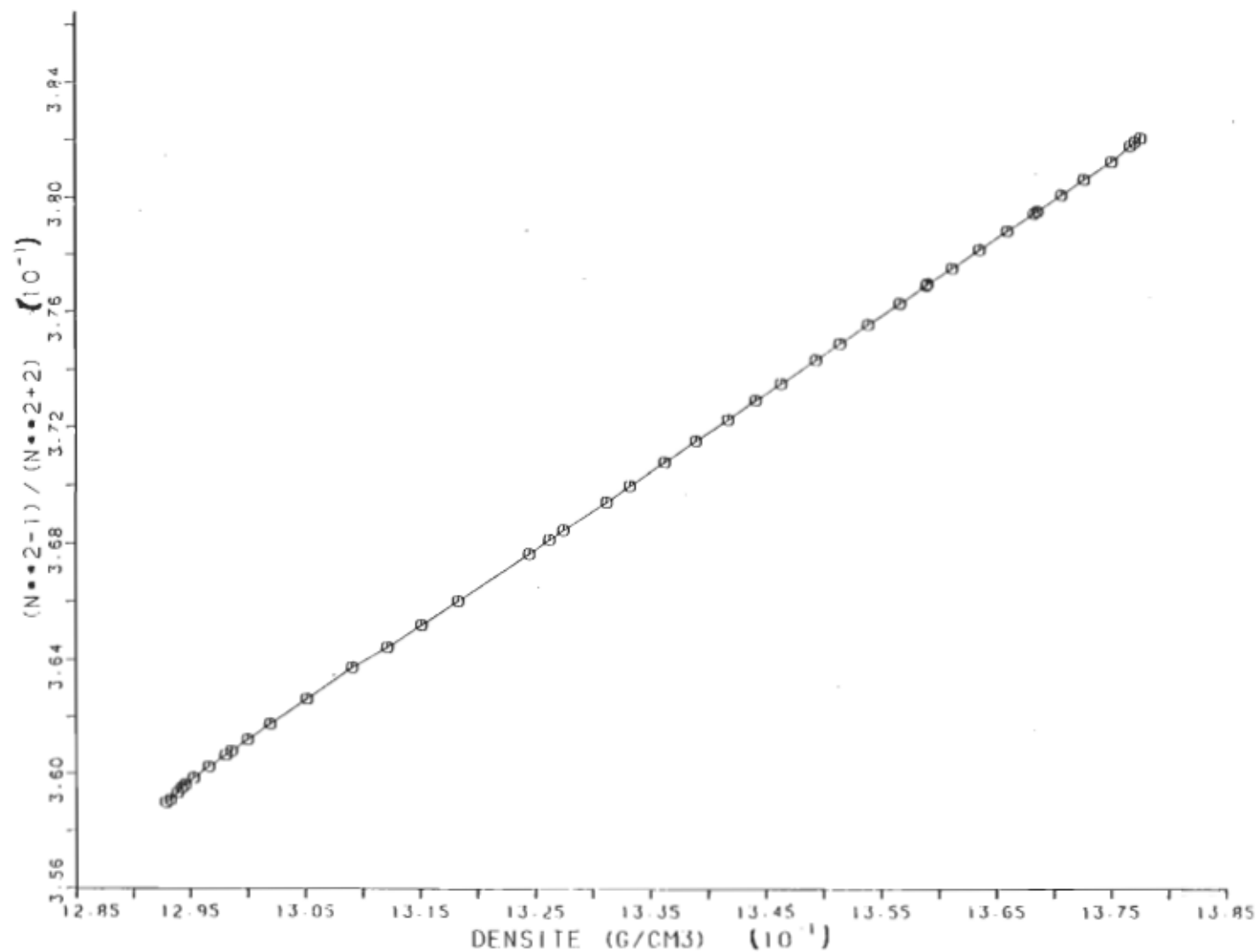
Figure (4.12): Courbe de l'équation de Lorentz-Lorenz L-L en fonction de la densité pour le liquide CS 2 à T=0,0 C.
