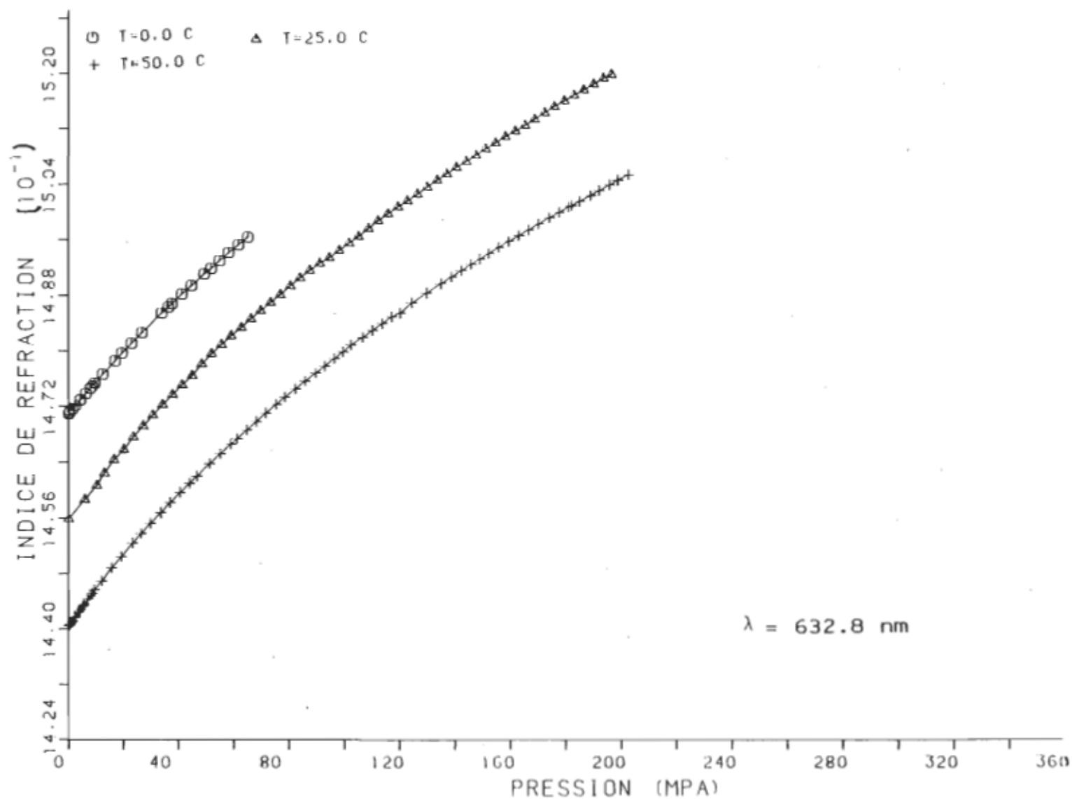
Figure (4.2): Courbe de l'indice de réfraction en fonction de la pression pour le \text{CCl}_4 à 0,0^\circ\text{C} , 25,0^\circ\text{C} et 50,0^\circ\text{C} .
