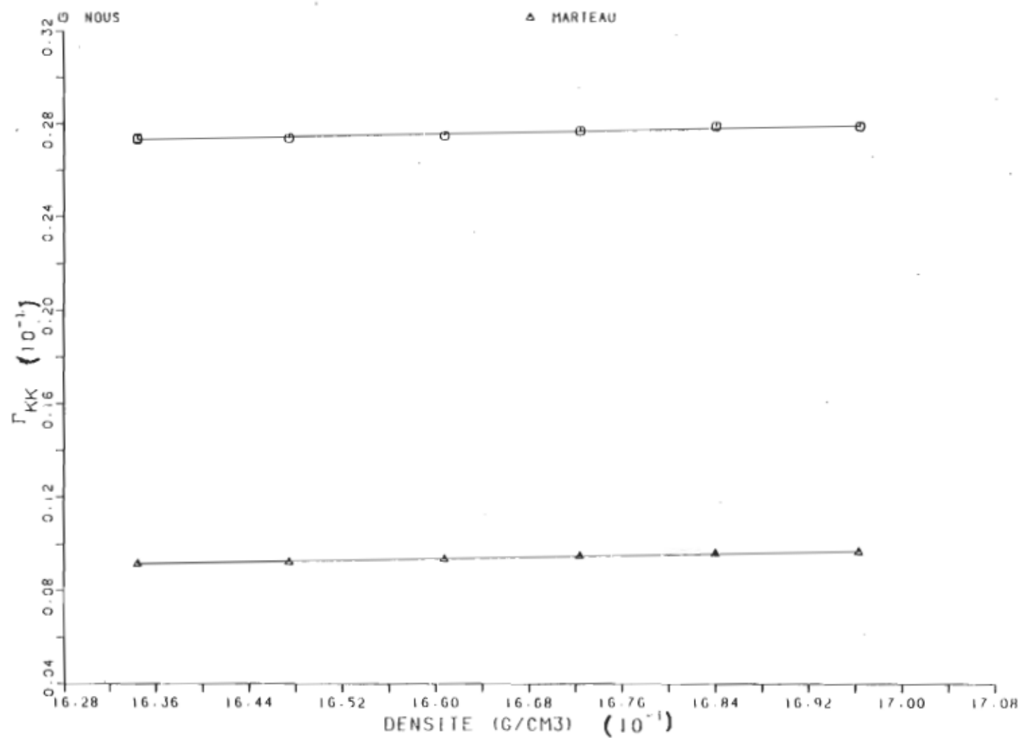
Figure (4.14): Courbe de \Gamma_{KK} en fonction de la densité pour le liquide \text{CCl}_4 à T = 0,0^\circ\text{C} .
