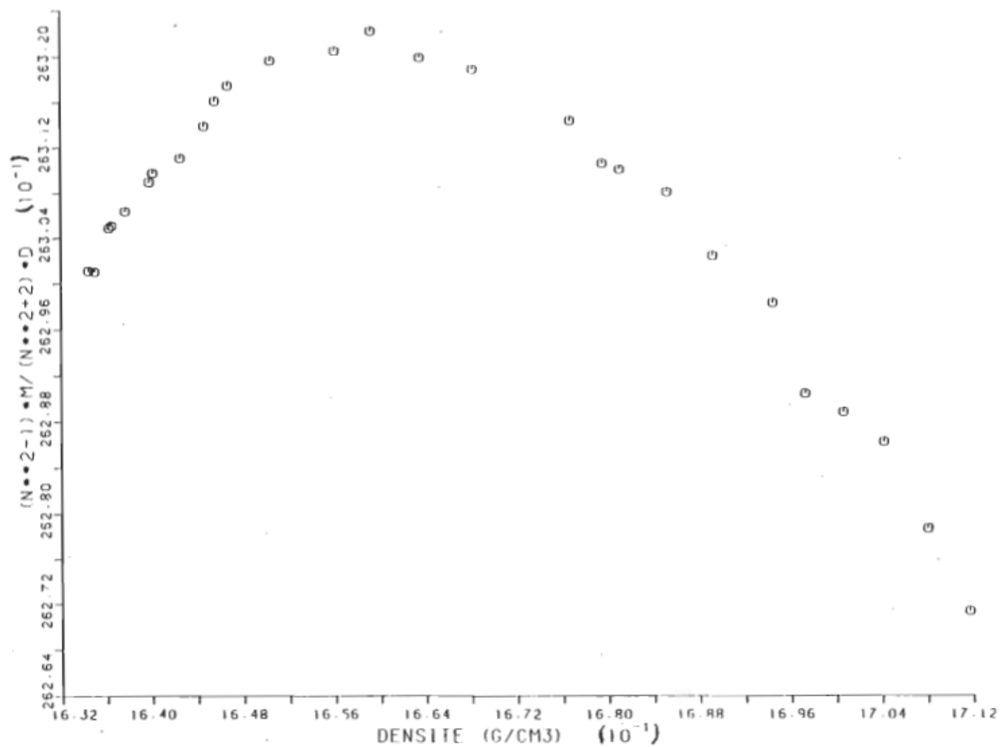
Figure (4.4): Courbe de l'équation de Lorentz-Lorenz modifiée L-L(m) en fonction de la densité pour le liquide \text{CCl}_4 à T=0,0^\circ\text{C} .
