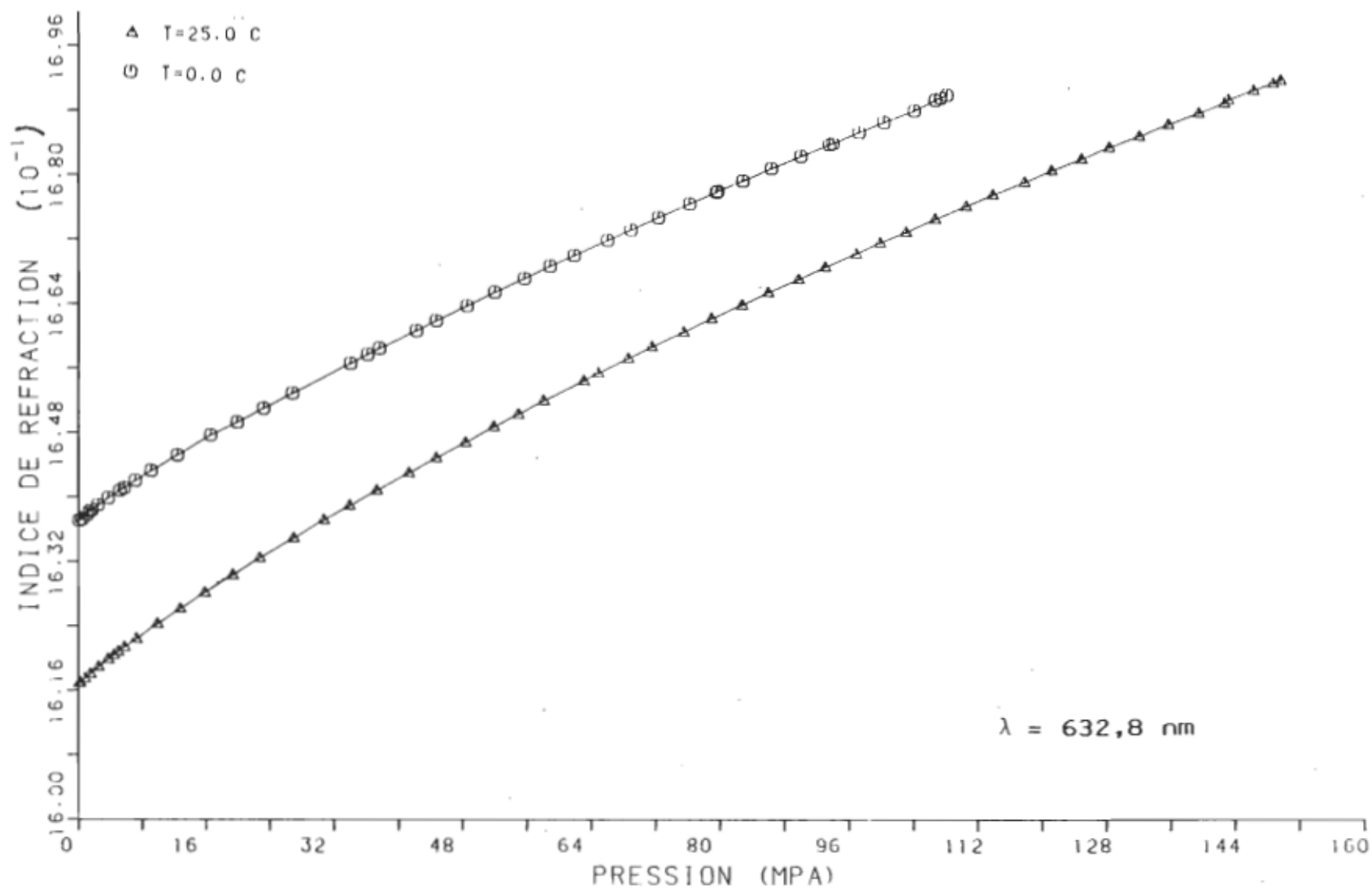
Figure (4.3): Courbe de l'indice de réfraction en fonction de la pression pour le liquide \text{CS}_2 à 0,0^\circ\text{C} et 25,0^\circ\text{C} .
