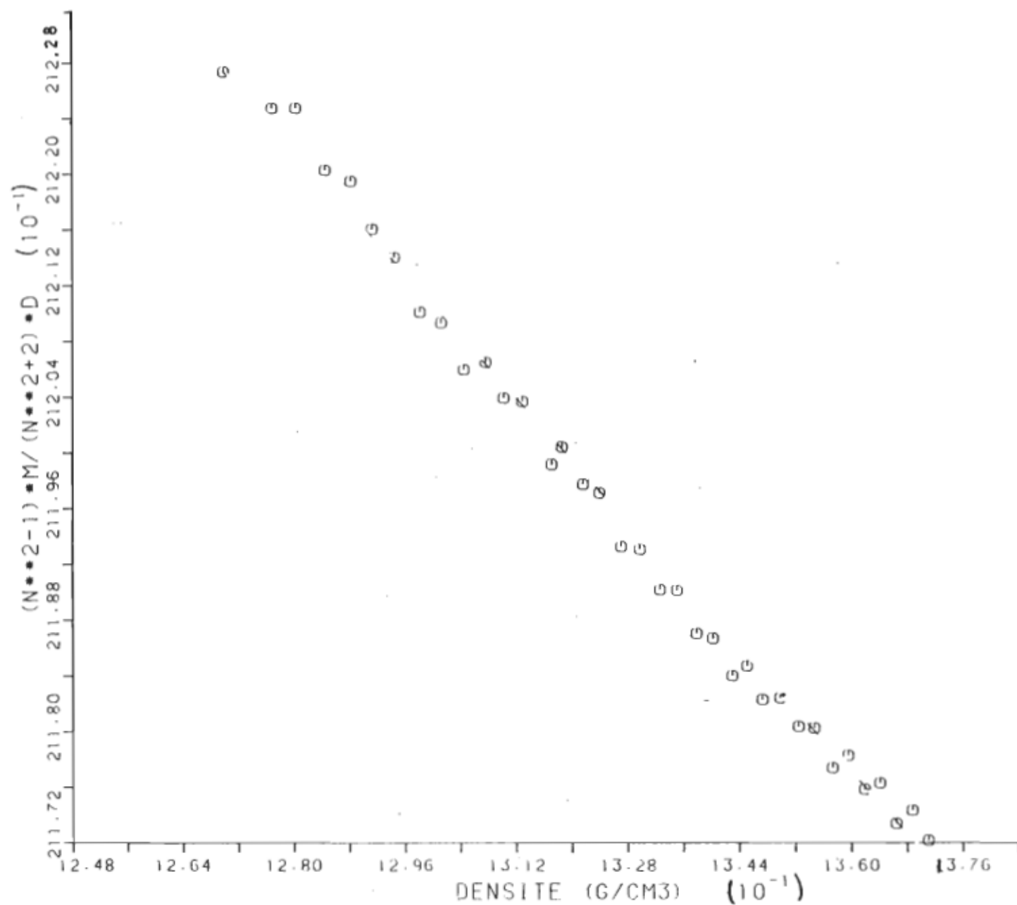
Figure (4.8): Courbe de l'équation de Lorentz-Lorenz modifiée L-L(m) en fonction de la densité pour le liquide CS 2 à T=25,0 C.
