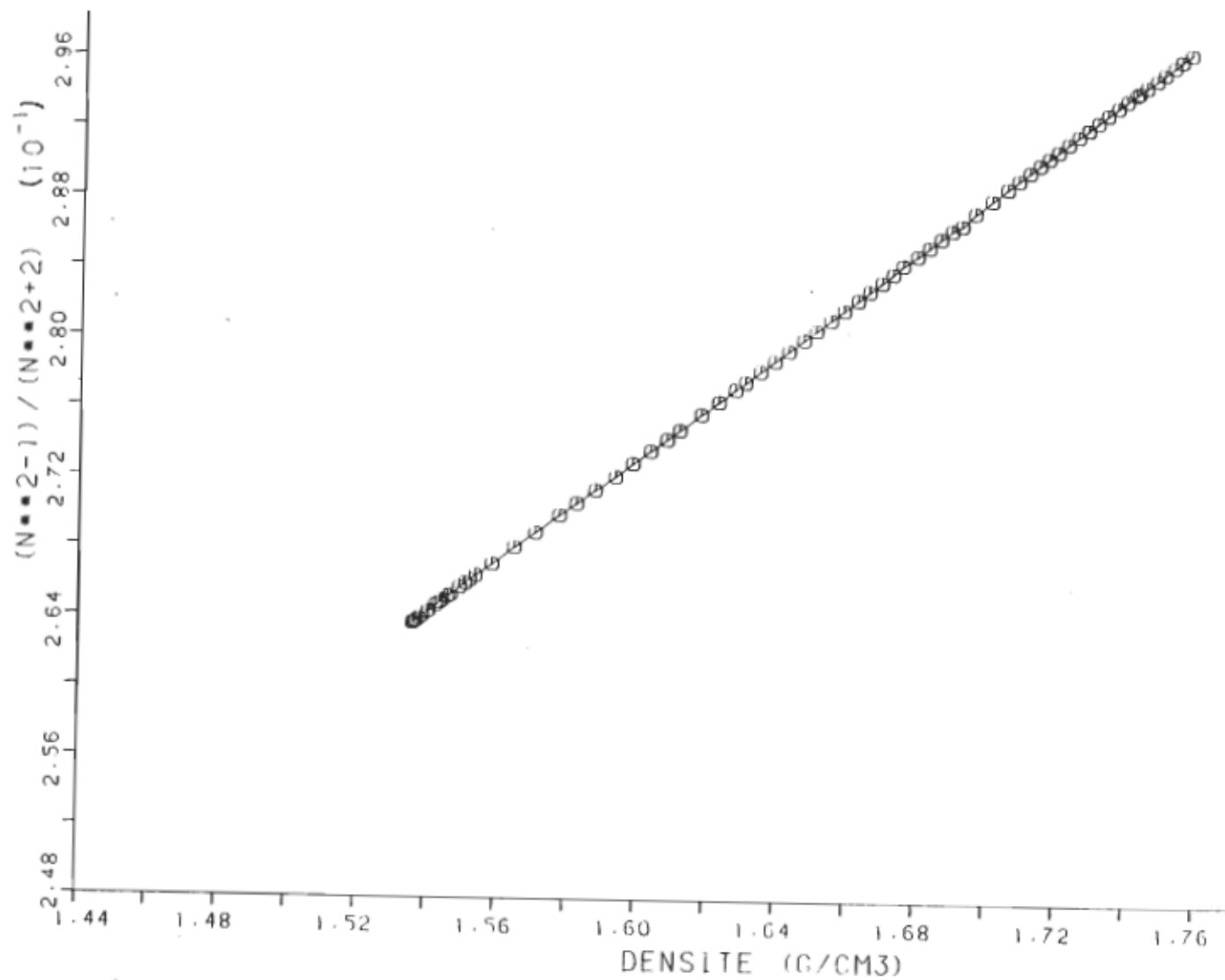
Figure (4.11): Courbe de l'équation de Lorentz-Lorenz L-L en fonction de la densité pour le liquide \text{CCl}_4 à T=50,0^\circ\text{C} .
