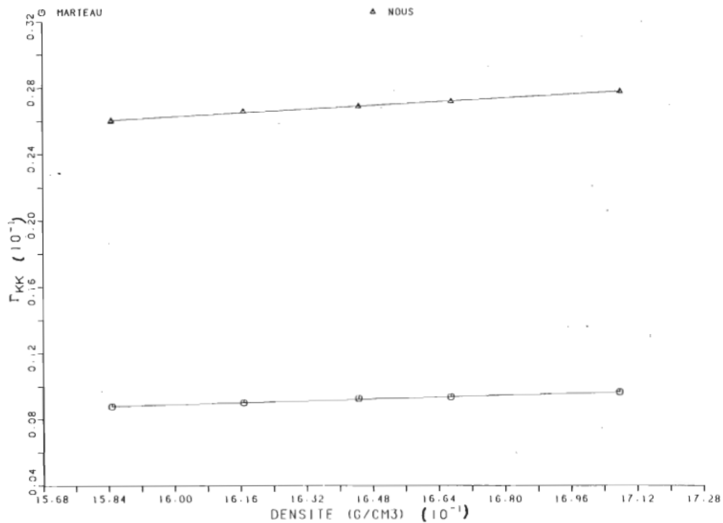
Figure (4.15): Courbe de \Gamma_{KK} en fonction de la densité pour le liquide \text{CCl}_4 à T = 25.0^\circ\text{C} .
