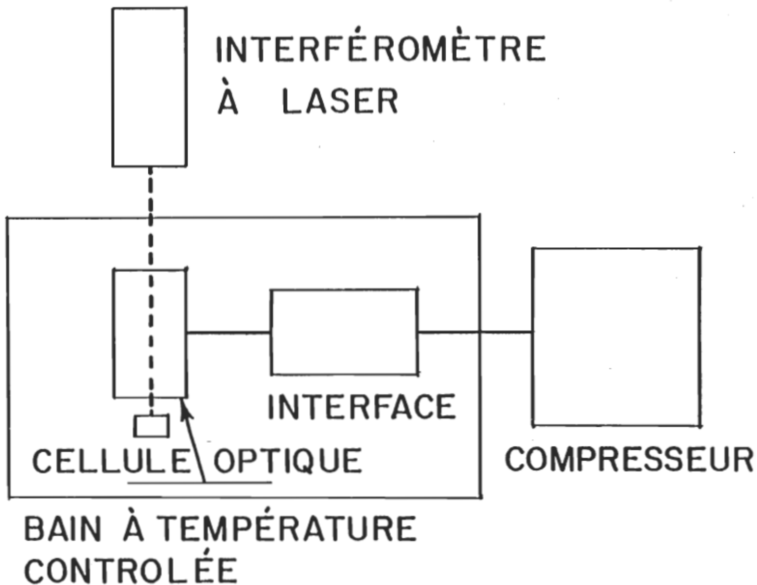
Figure (3.1): Système pour la mesure de propriétés piézo-optiques des liquides
