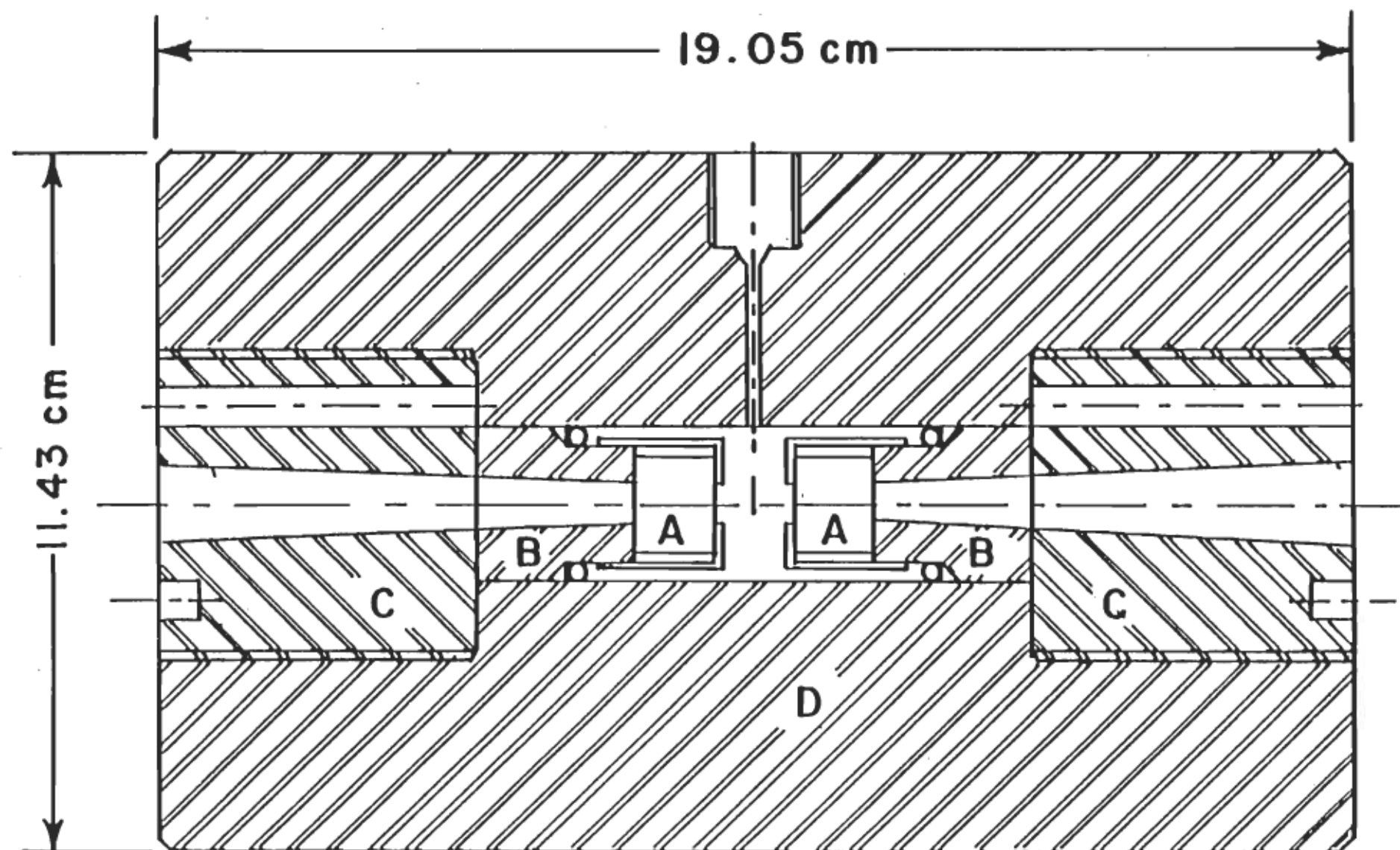
Figure(3.4): Coupe de la cellule optique pour les liquides.
