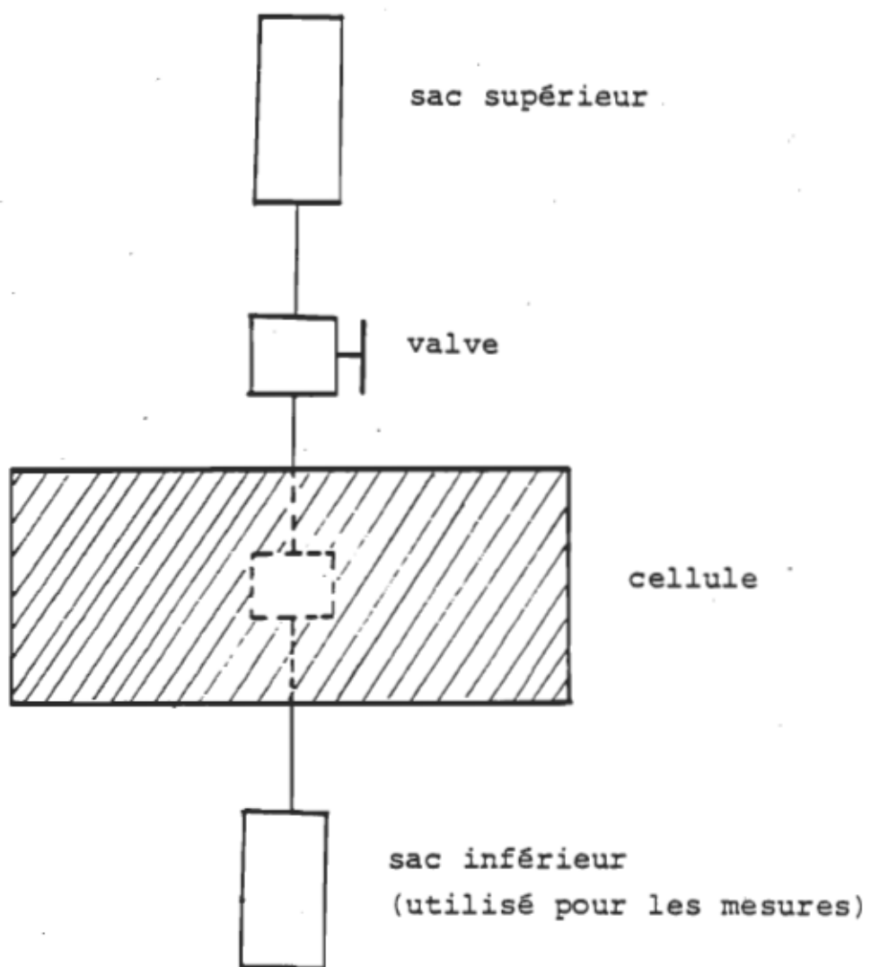
Figure (4.1) : Le système utilisé pour enlever les bulles d'air
