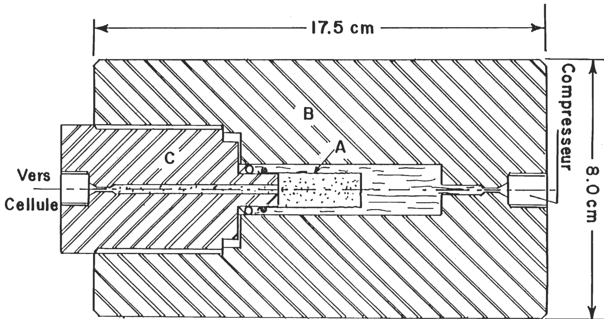
Figure(3.5) : Coupe de l'interface; ---:huile de compression ....liquide à étudier.
