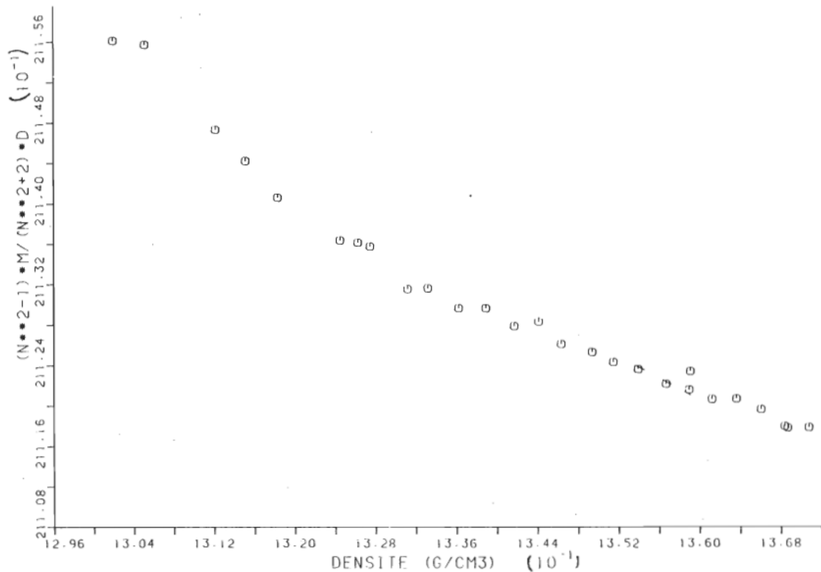
Figure (4.7): Courbe de l'équation de Lorentz-Lorenz modifiée L-L(m) en fonction de la densité pour le liquide \text{CS}_2 à T=0,0^\circ\text{C} .
