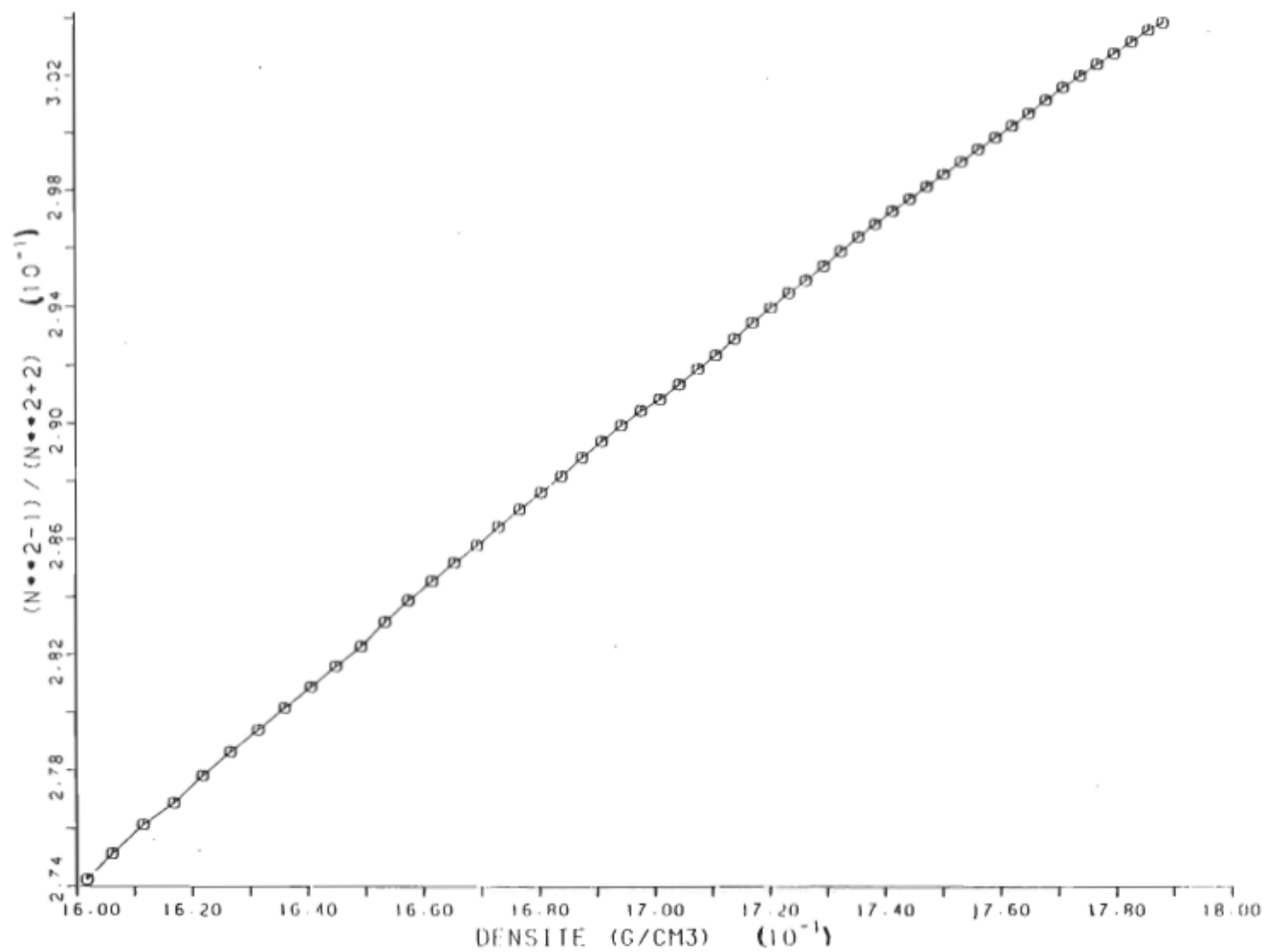
Figure (4.10): Courbe de l'équation de Lorentz-Lorenz L-L en fonction de la densité pour le liquide \text{CCl}_4 à T=25,0\text{ }^\circ\text{C} .
