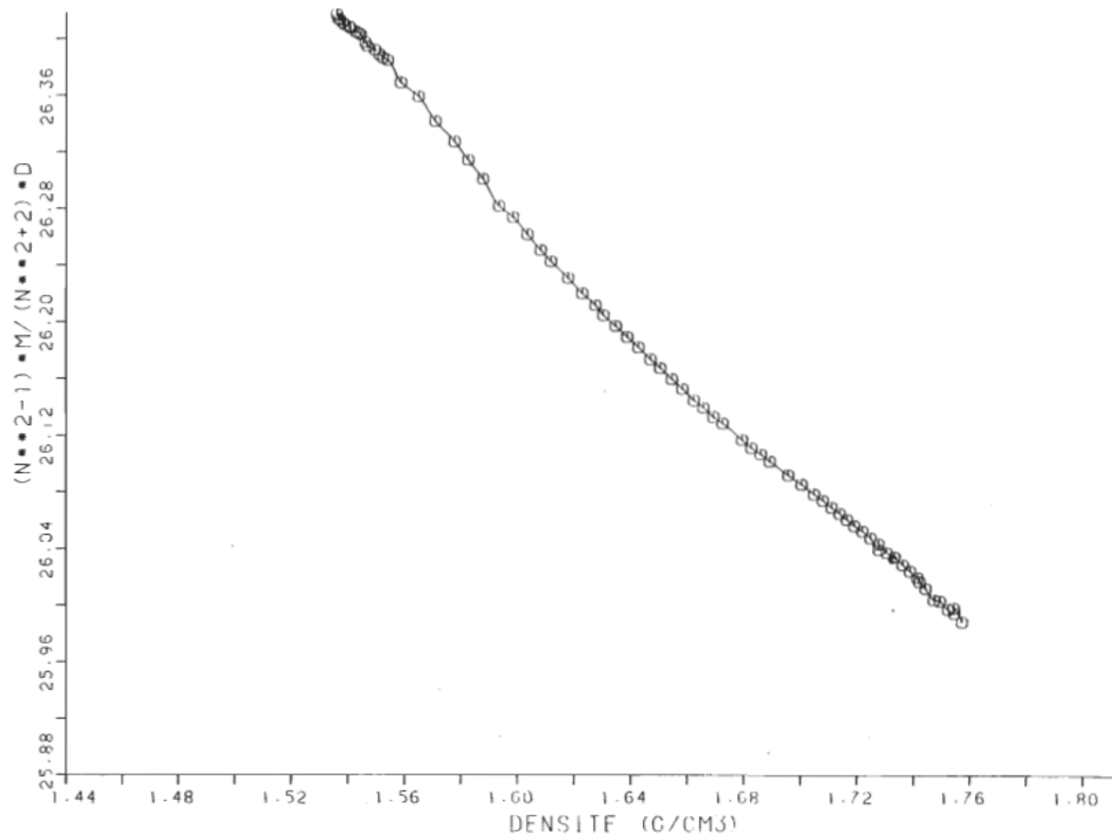
Figure (4.6): Courbe de l'équation de Lorentz-Lorenz modifiée L-L(m) en fonction de la densité pour le liquide CCl 4 à T=50,0 °C.
