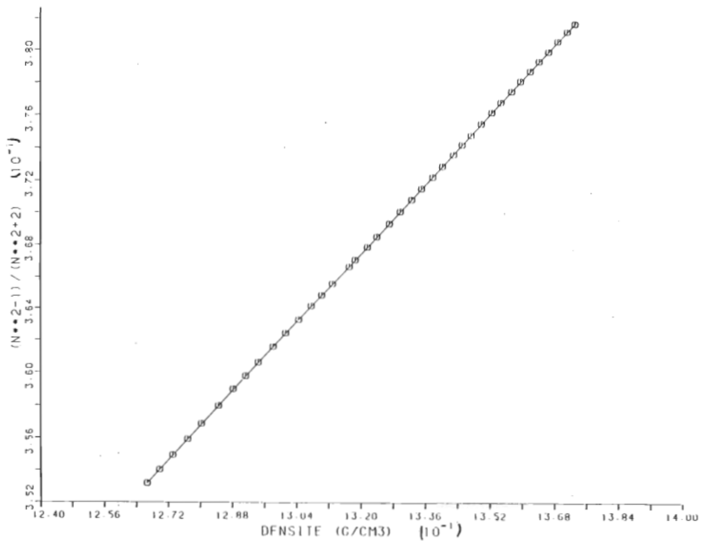
Figure (4.13): Courbe de l'équation de Lorentz-Lorenz L-L en fonction de la densité pour le liquide CS 2 à T=25,0°C.
