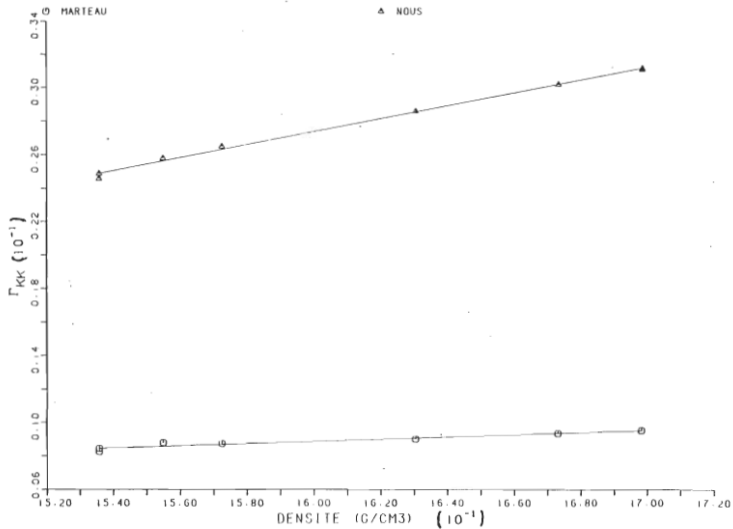
Figure (4.16): Courbe de \Gamma_{KK} en fonction de la densité pour le liquide \text{CCl}_4 à T = 50,0^\circ\text{C} .
