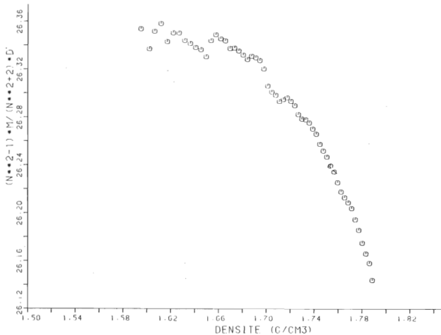
Figure (4.5): Courbe de l'équation de Lorentz-Lorenz modifiée L-L(m) en fonction de la densité pour le liquide \text{CCl}_4 à T=25,0^\circ\text{C} .
