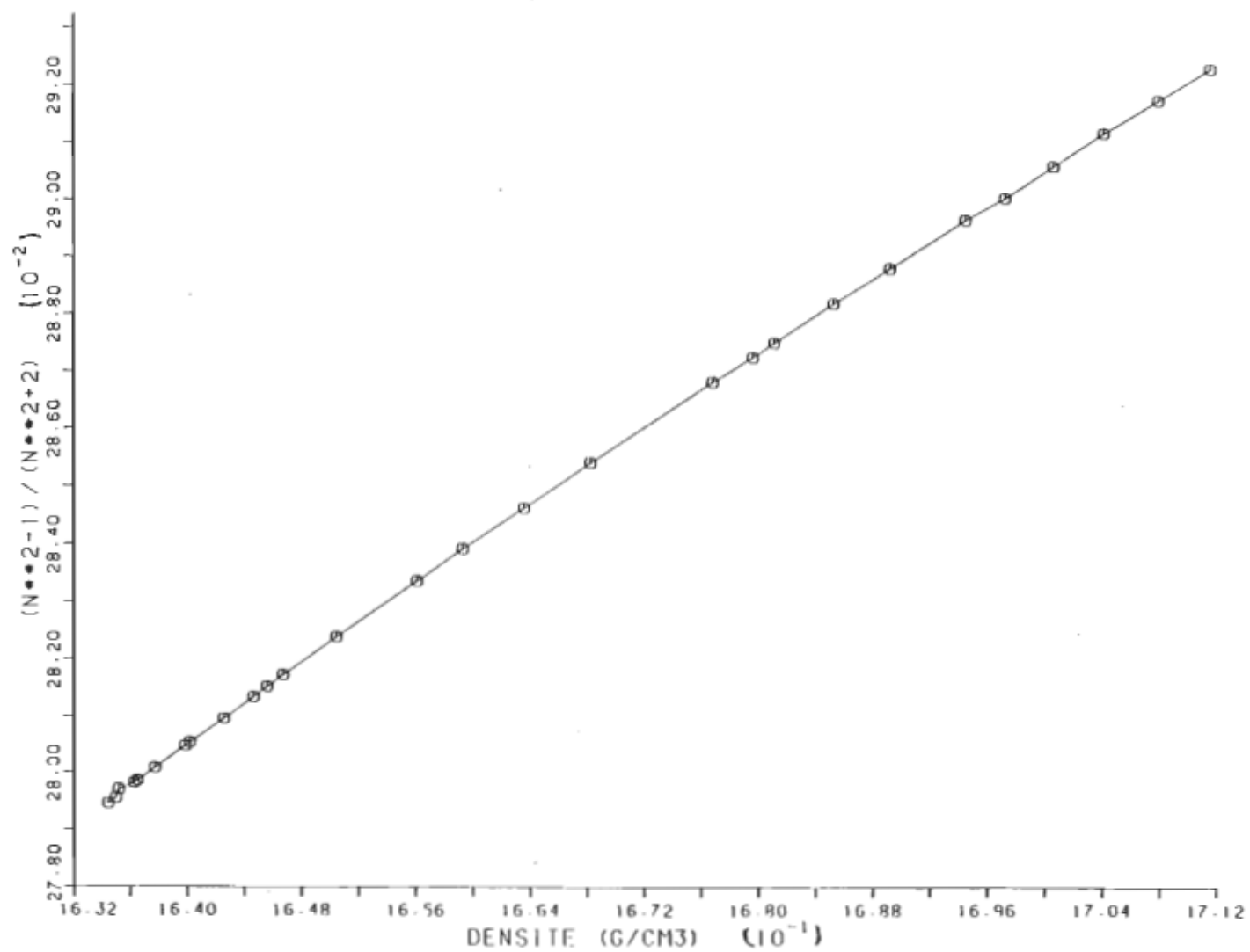
Figure (4.9): Courbe de l'équation de Lorentz-Lorenz L-L en fonction de la densité pour le liquide CCl 4 à T=0,0 C.
