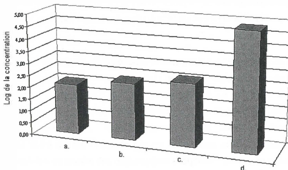
FIGURE 1.6. Logarithme de la concentration (mg/g) minimum de produit appliqué induisant 100% de mortalité chez les larves de Galleria mellonella . Dans le graphique ci haut, sont identifié par les lettres les produits suivants; a. 2,3-époxy-propan-1-ol, b. 4,5-époxy-pentan-2-ol, c. 1,3-(bis (2,3-époxypropoxy)-propan-2-ol) et d. l'huile de neem.
